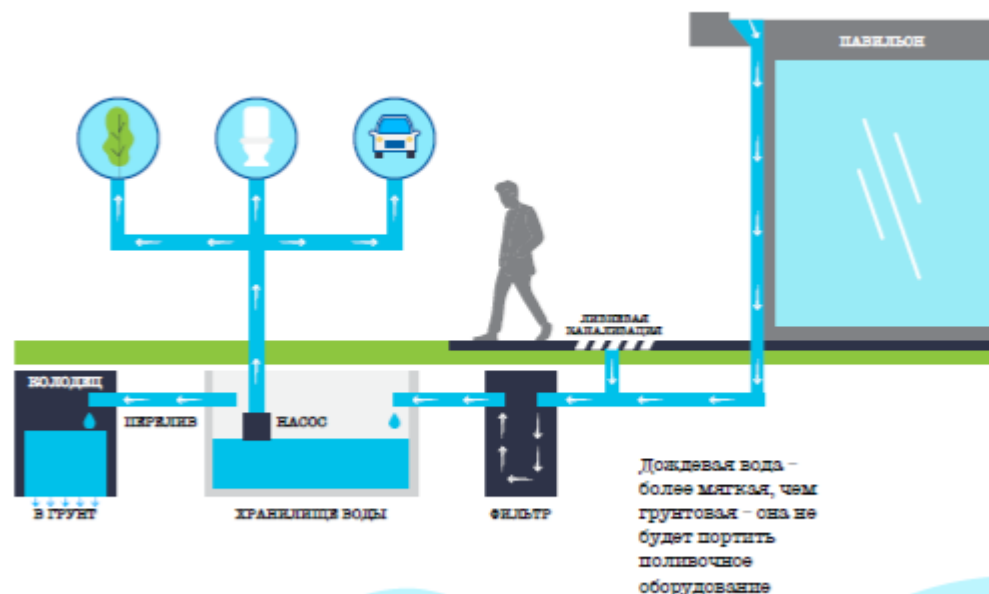
СХЕМА ПРОЕКТНОГО РЕШЕНИЯ ПО СБОРУ И УТИЛИЗАЦИИ ВОДЫ
